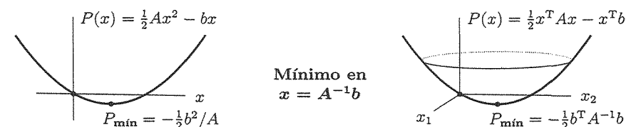
Figura 6.4 La gráfica de una cuadrática positiva P(x) es un tazón parabólico.
