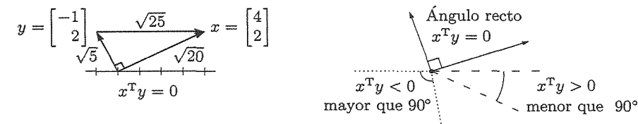
Figura 3.2 Triángulo rectángulo con 5 + 20 = 25 . Ángulo con línea punteada 100^\circ , ángulo con línea discontinua 30^\circ .
