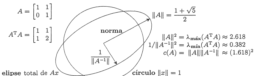
Figura 7.1 Las normas de A y A^{-1} provienen de la Ax más larga y más corta.
