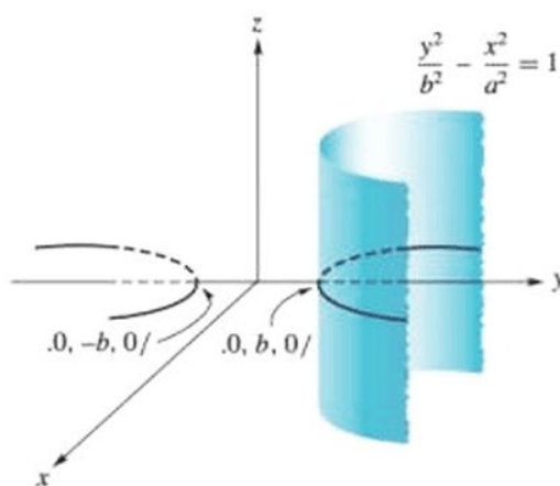
Figura 8.14 ▲ Cilindro hiperbólico
