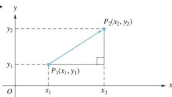
Figura 4.10 ►
