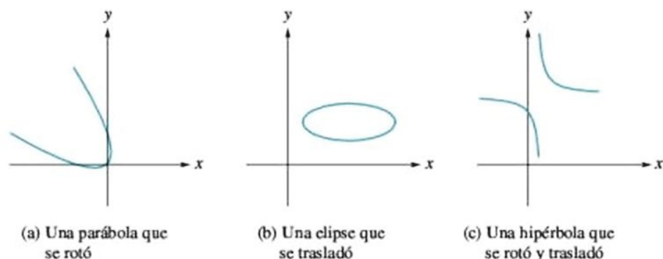
Figura 8.4 ►
