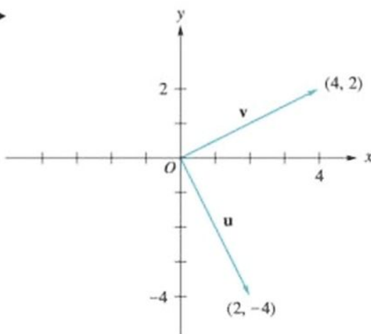
Figura 4.24 ► Vectores ortogonales
