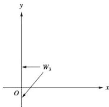
Figura 6.3 ▲
