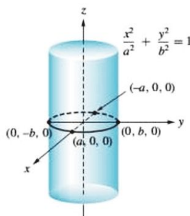
Figura 8.9 ▲ Cilindro elíptico
