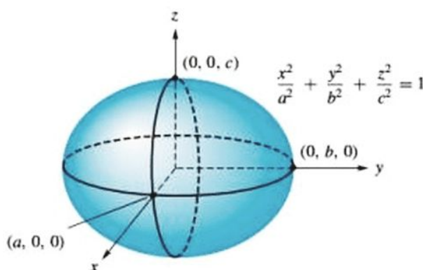
Figura 8.7 ▲ Elipsoide
