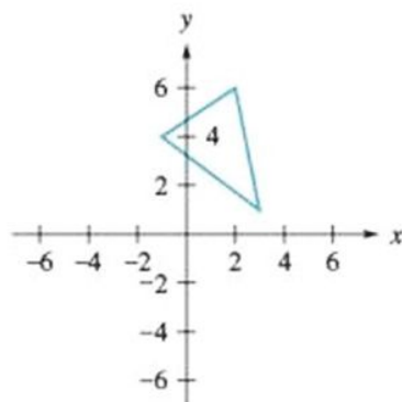
Figura 4.12 ▲
