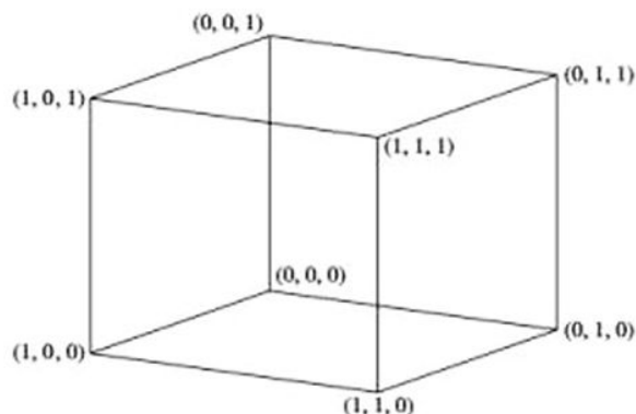
Figura 4.38 ▲
