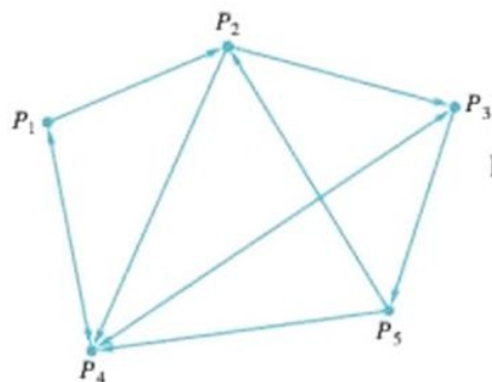
Figura 2.11 ▲
