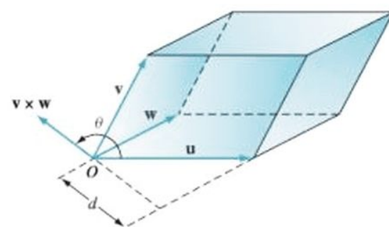
Figura 5.5 ►
