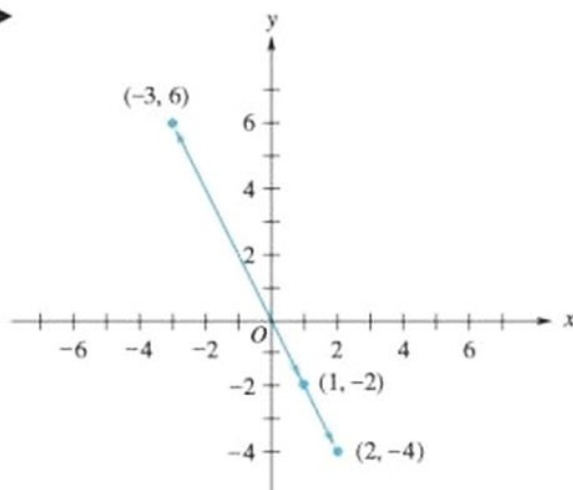
Figura 4.18 ►
