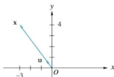
Figura 4.25 ▲
