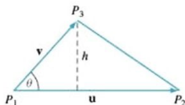
Figura 5.3 ▲
