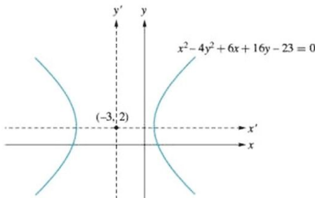
Figura 8.5 ►
