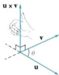
Figura 5.2 ▲
