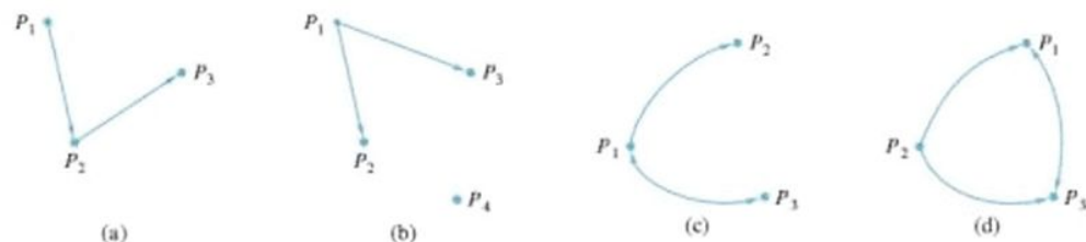
Figura 2.1 ►
