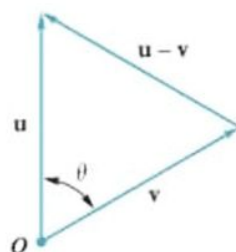
Figura 4.22 ▲
