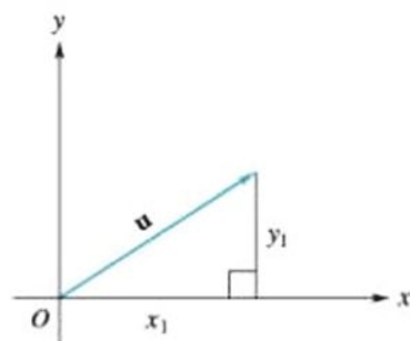
Figura 4.9 ▲
