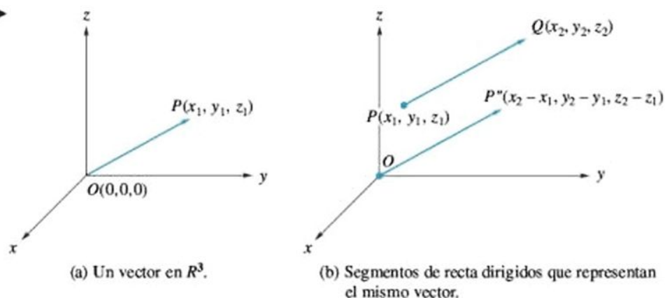
Figura 4.31 ►
