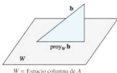
Figura 6.17 ▲
