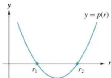
Figura 4.34 ▲
