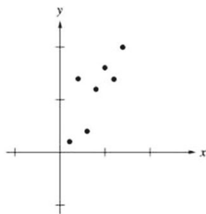
Figura 1.10 ▲
