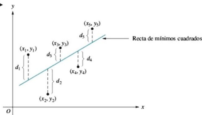
Figura 6.19 ►
