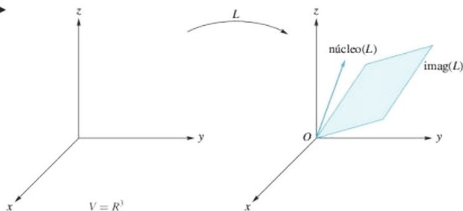
Figura 9.2 ►
