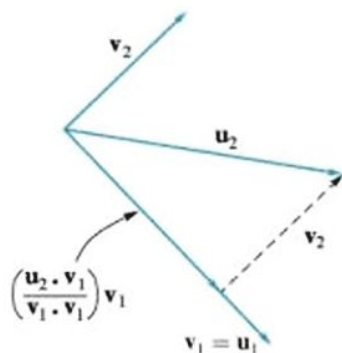
Figura 6.13 ▲
