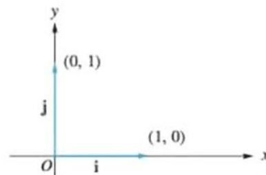
Figura 4.26 ▲ Vectores ortogonales
