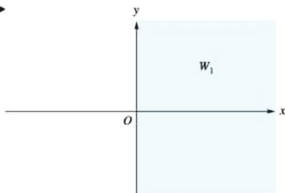
Figura 6.1 ►
