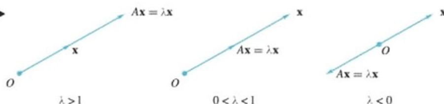
Figura 7.2 ►
