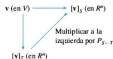
Figura 6.12 ▲
