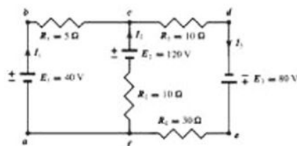
Figura 2.13
