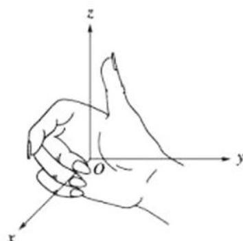
Figura 4.28 ▲
