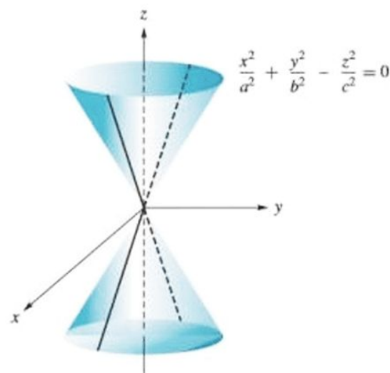
Figura 8.11 ▲ Cono
