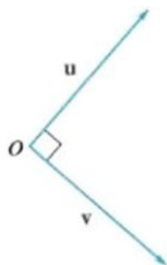
Figura 4.23 ▲ Vectores ortogonales
