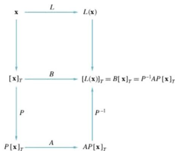
Figura 9.4 ►
