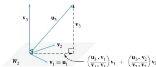
Figura 6.14 ►
