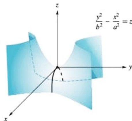
Figura 8.13 ▲ Paraboloide hiperbólico
