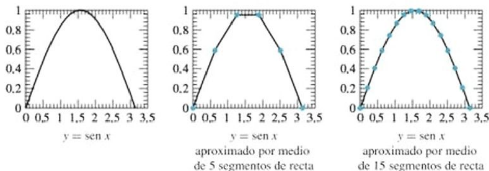
Figura B
