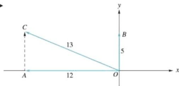
Figura 4.20 ►
