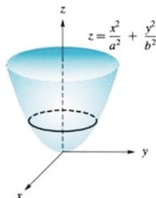
Figura 8.8 ▲ Paraboloide elíptico
