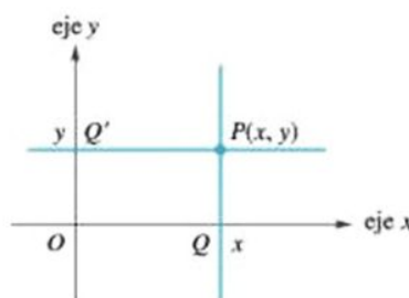
Figura 4.4 ▲
