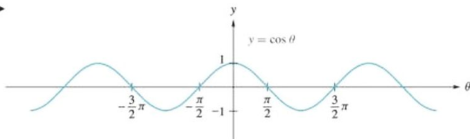
Figura 4.35 ►
