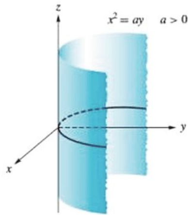
Figura 8.15 ▲ Cilindro parabólico
