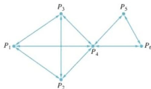
Figura 2.7 ▲
