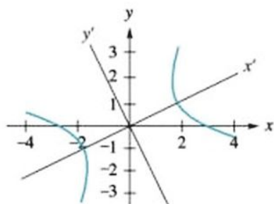
Figura B
