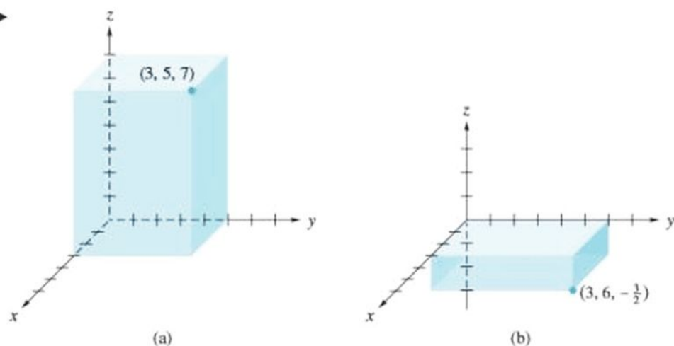
Figura 4.30 ►
